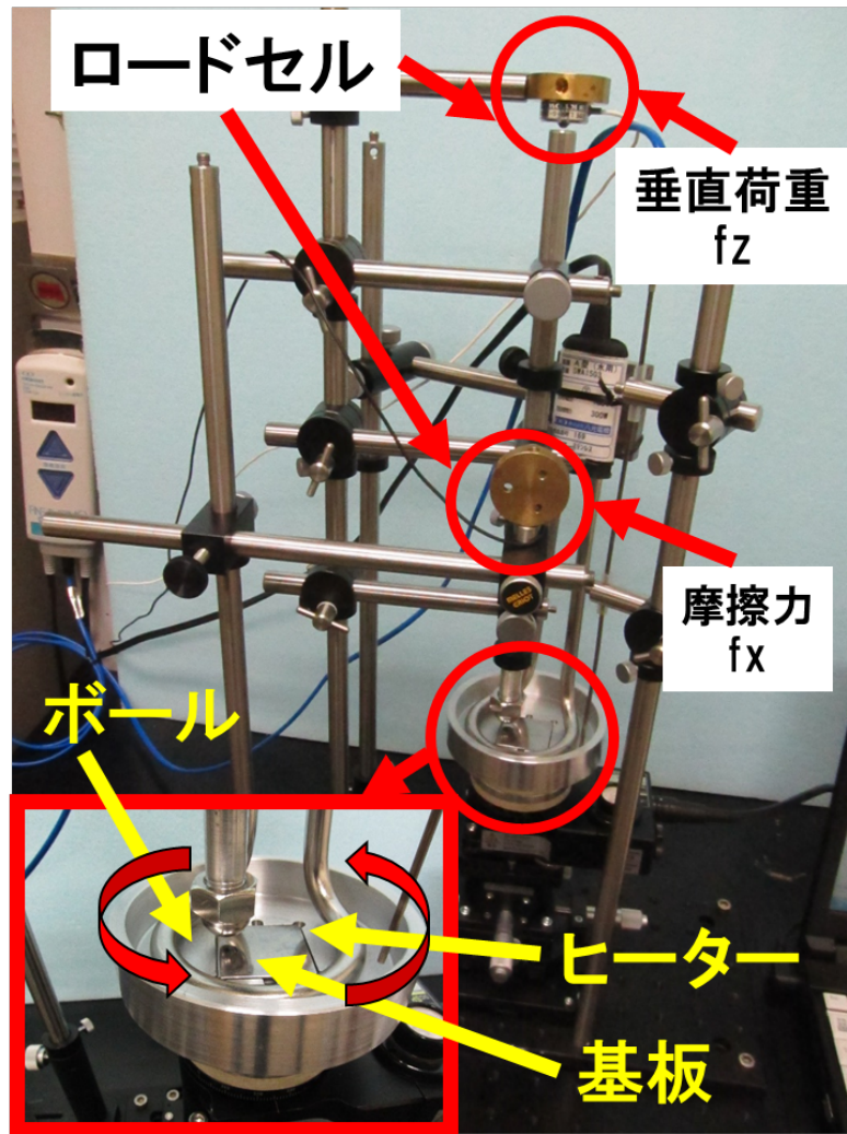
成膜装置(摩擦試験機)
